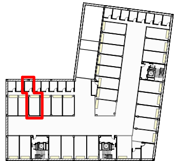
2 Localización garaje/trastero 1 : 1000
