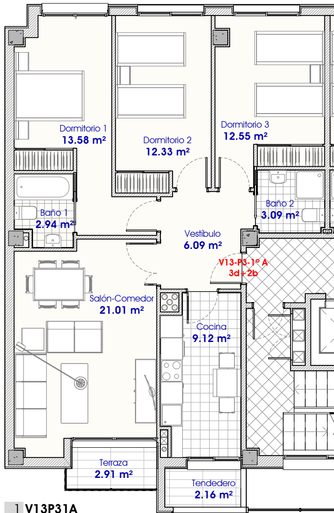
1 V13P31A 1 : 100
