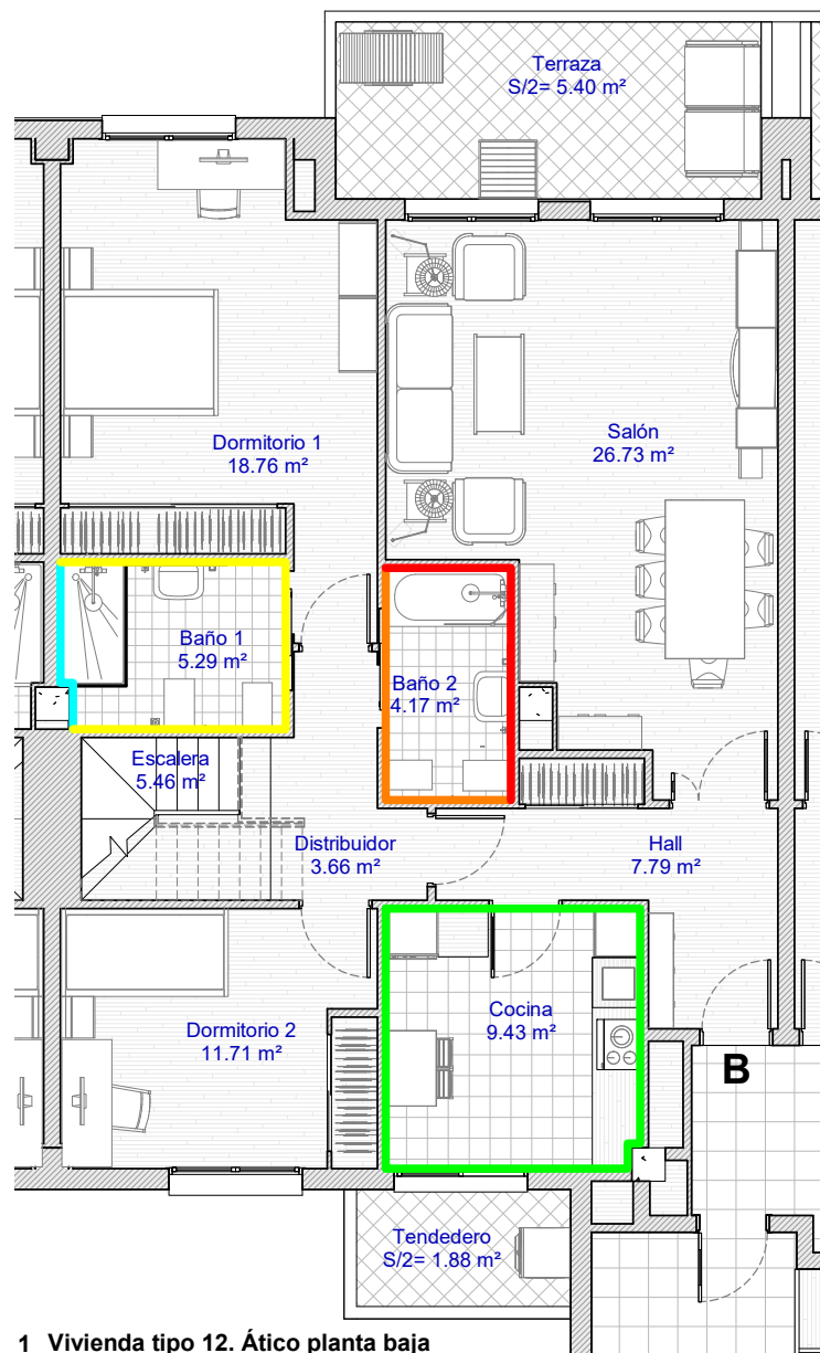
1 Vivienda tipo 12. Ático planta baja 1 : 100
